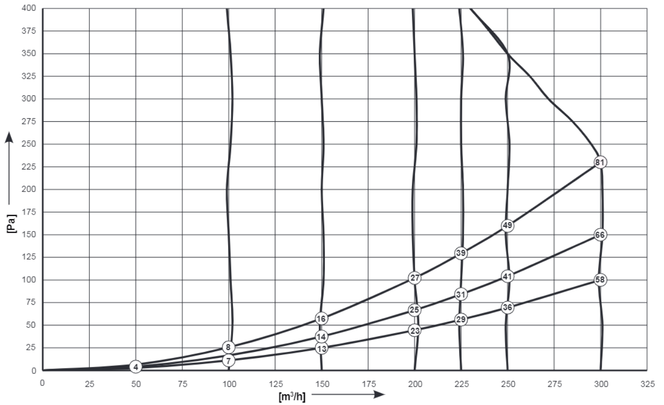
Fan graph Renovent Sky 300
