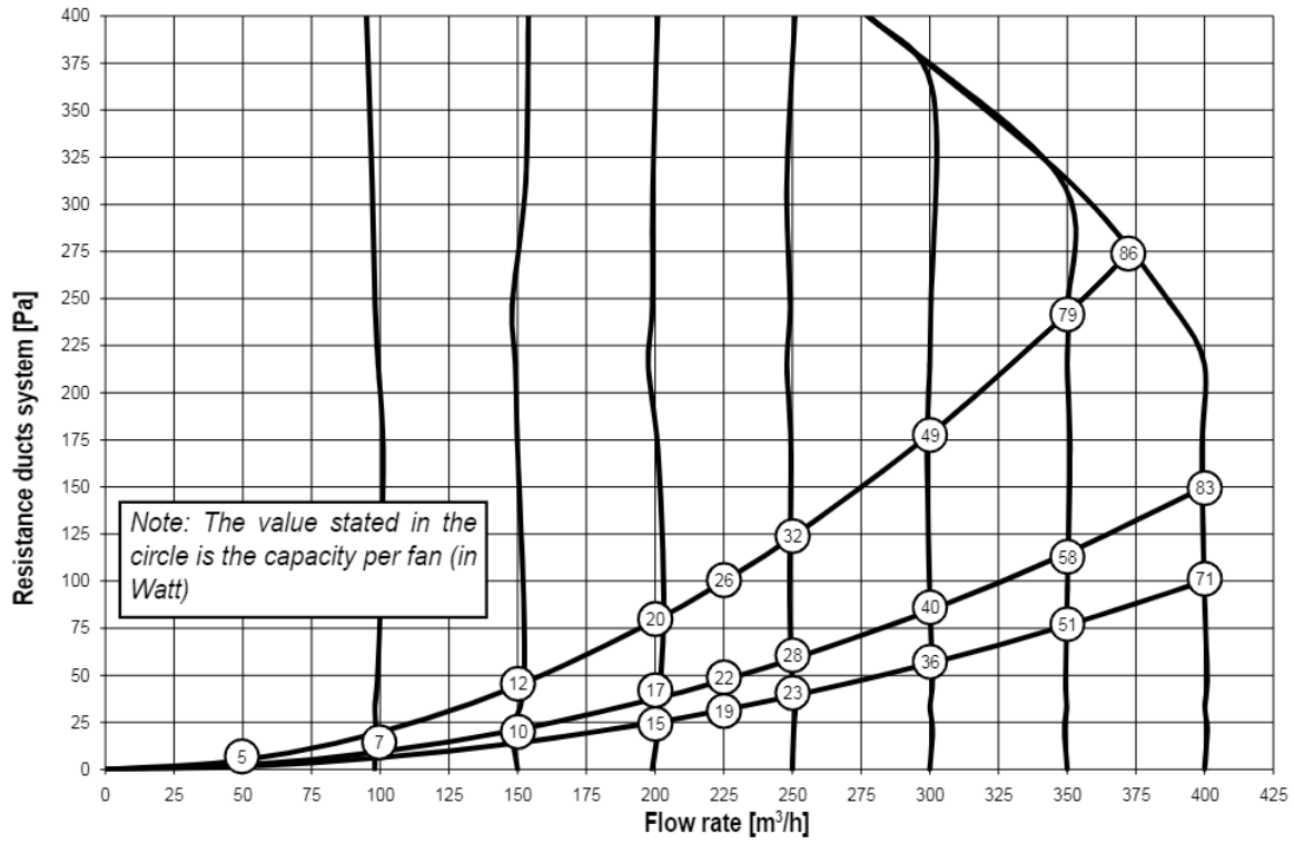
Fan graph Renovent Excellent 400
